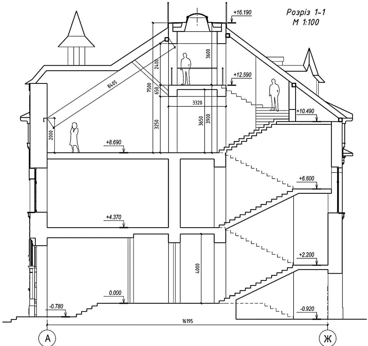
Рис.1. Поперечний переріз будівлі
